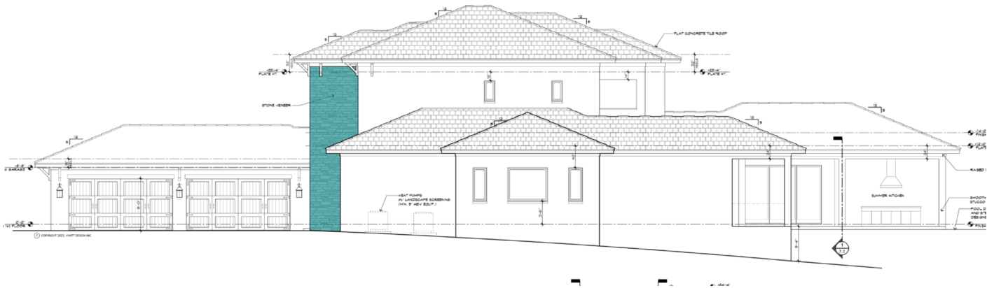
Right Elevation
